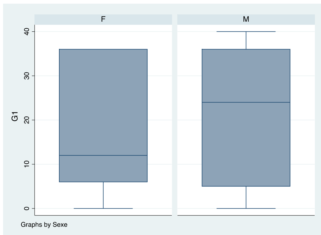
Graphique 1 : Distribution de la durée de chômage des diplômés de Licence, par sexe
