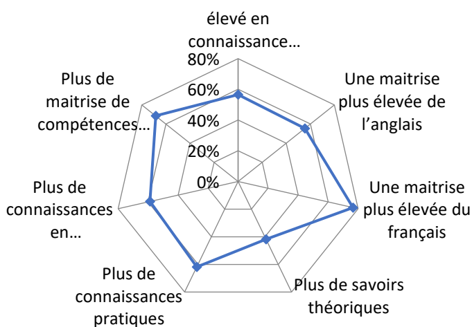
Graphique 30: Indices d'amélioration perçus par les ingénieurs de l'Université de Sfax
